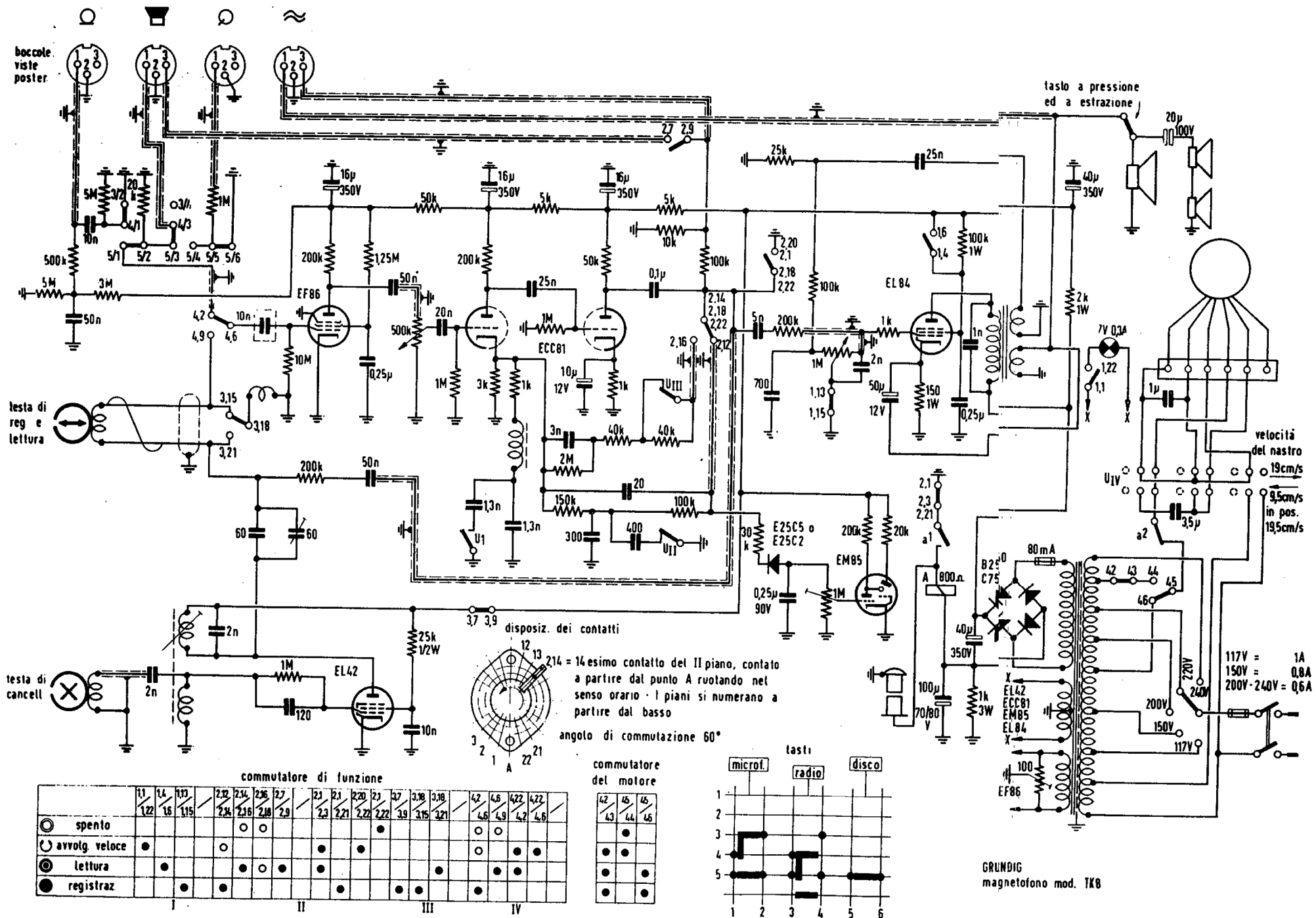
Schema elettrico del magnetofono Grundig, mod. TK 8
